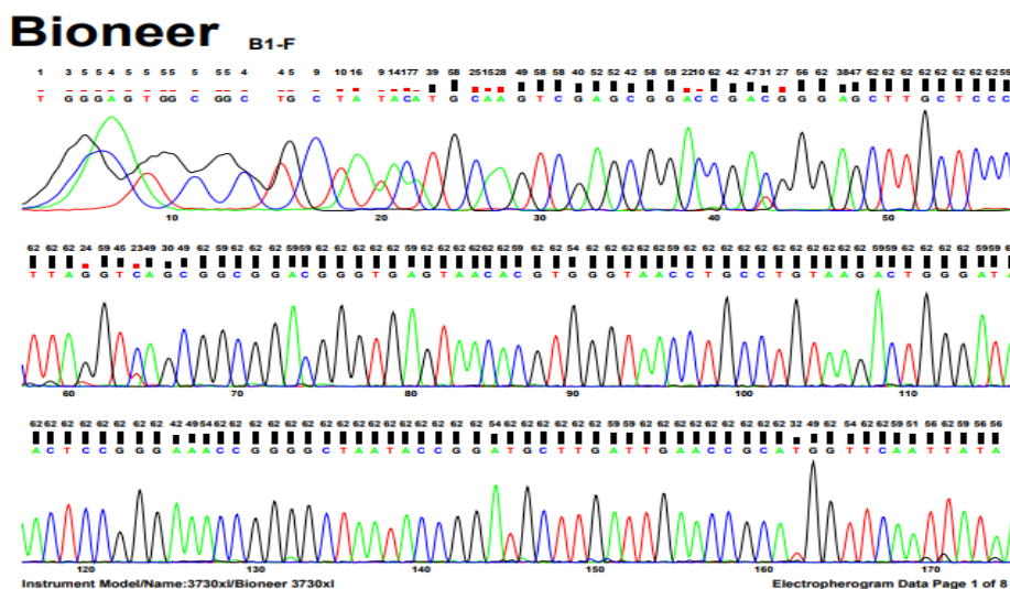
شکل ۹: نتیجه سکانسینگ و بلاست pspC Forward
