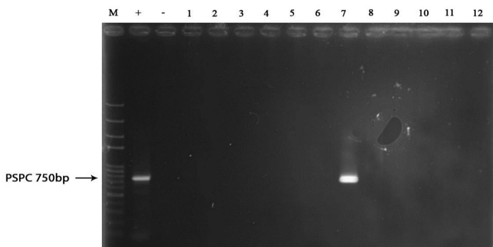
شکل ۲: نتیجه PCR ژن های pspC
