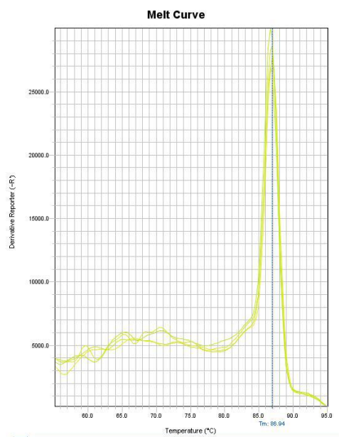
شکل ۷: نتایج منحنی ذوب Real time PCR
