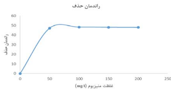
نمودار ۷: تأثیر غلظت یون منیزیم بر روی عمل جذب با استفاده از پامیس خام (۵ g)
