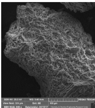
شکل ۲: SEM پامیس اصلاحی قبل از جذب سفالکسین (با بزرگنمایی ۶۴۰*)
