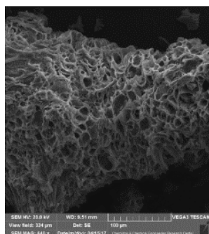
شکل ۴: SEM پامیس اصلاحی بعد از جذب سفالکسین ( با بزرگنمایی ۶۴۰*)
