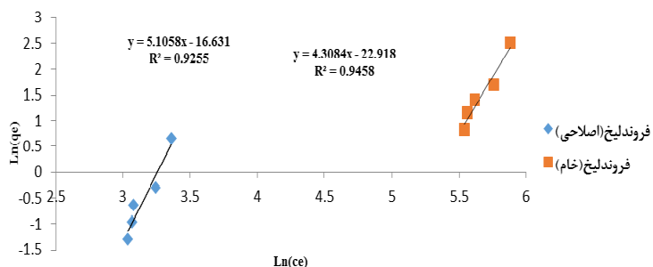
نمودار ۱۲: ایزوترم فرندلیخ
