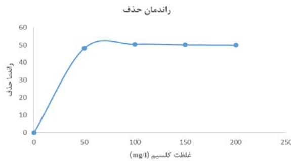
نمودار ۶: تأثیر غلظت یون کلسیم بر روی عمل جذب با استفاده از پامیس خام (۵ g)
