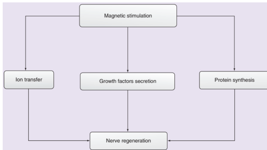
شکل ۴- ساز و کار عملکرد تحریک میدان مغناطیسی بر بازسازی اعصاب ۲۹
